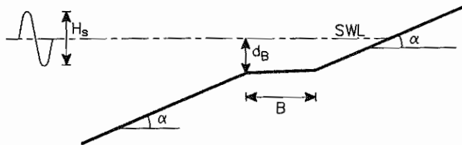
Figure 2 Berm parameters
